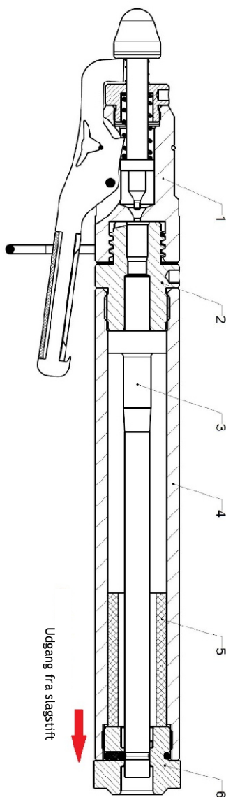
Fig. : Bullen Blitz- boltanordning (ikke ladet og afspændt)
