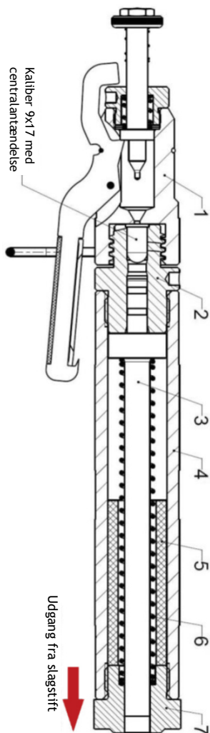
Fig. : Blitz Kerner- boltanordning (ladt og spændt)
